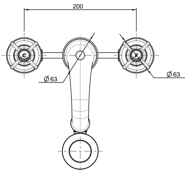
- Schema di foratura consigliato / Recommended drilling scheme
